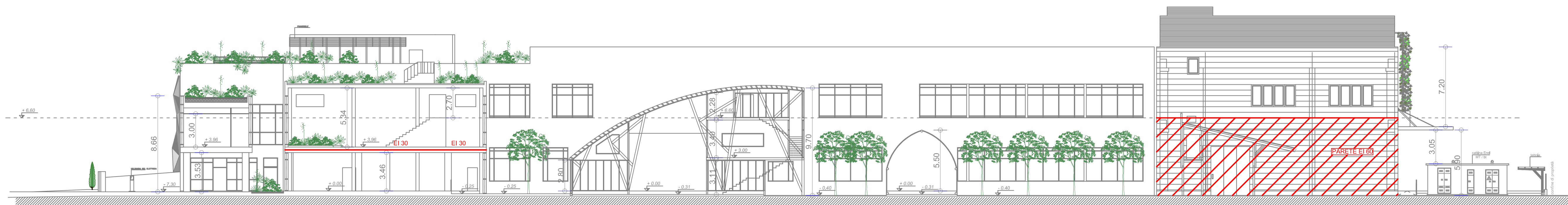
SEZIONE B-B
